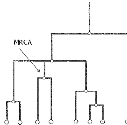
Afb. 5: Voorstelling van een evolutionaire boom waarbij de grijze bollen verschillende individuen of populaties voorstellen. MRCA is de meest recente voorouder van de 2 afgesplitste takken
